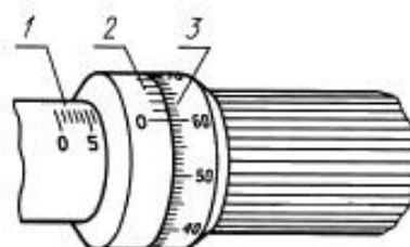
Черт. 8
