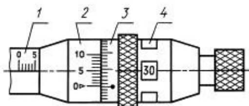
Черт. 7
