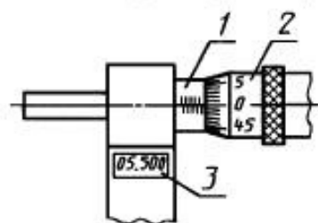
Цифровое устройство микрометров типов МВМЦ, МВТЦ, МВПЦ
