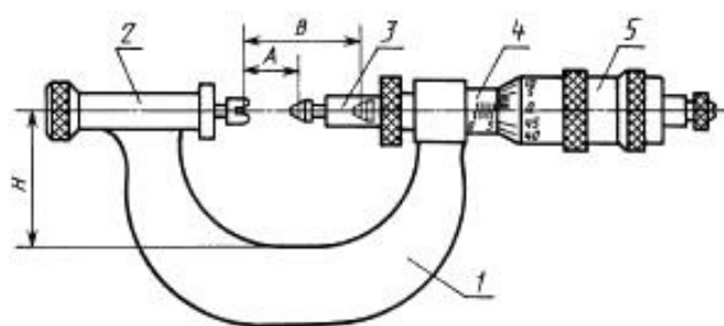
Микрометры типов МВМ, МВТ, МВП
