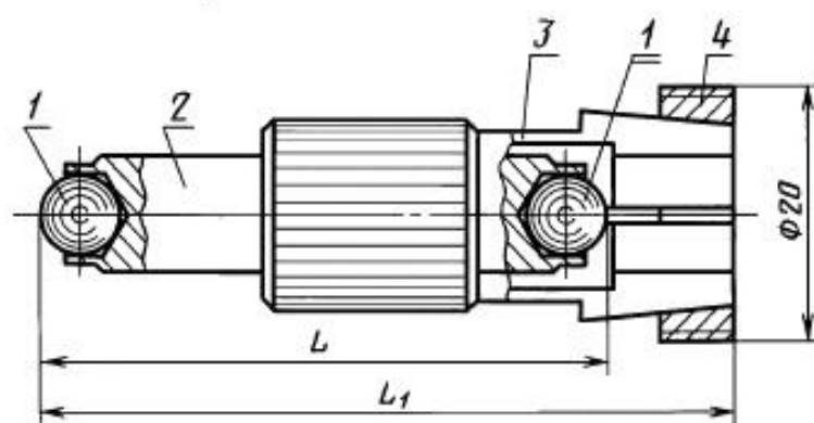
Приспособление с дополнительной пяткой
