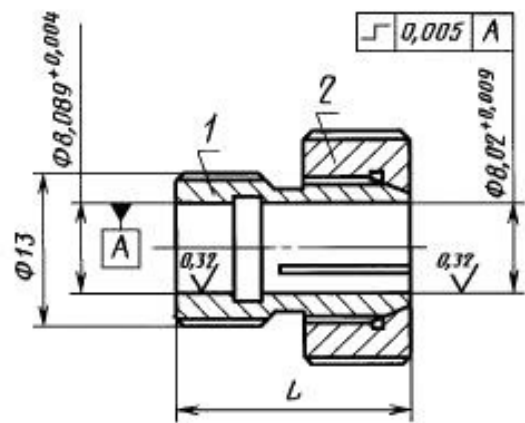
1 — втулка; 2 — гайка
